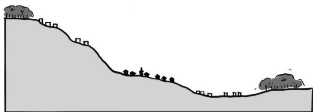
Coupe schématique d'un bourg de piedmont - Bourg de Murat (© Journal La Montagne « Ce qui fait de Murat (Cantal), une petite cité de caractère » 8-09-2018)
