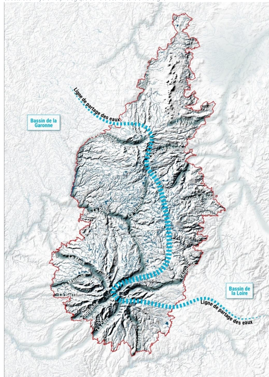
Structuration hydromorphologique du Parc des Volcans d'Auvergne
