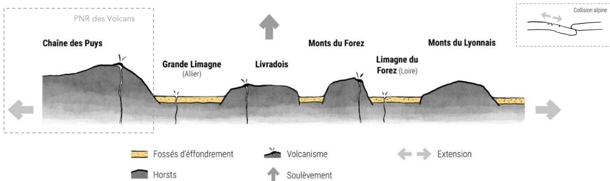
Coupe géologique synthétique illustrant les conséquences de la collision entre les plaques Européenne et Africaine – Source : Guide du relief du Massif central, Henri Widmer, Ed. GAP
