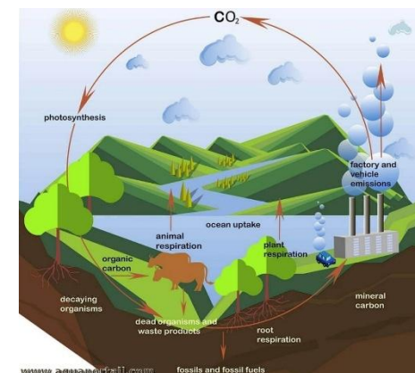
www.aquaportail.com Cycle du carbone
